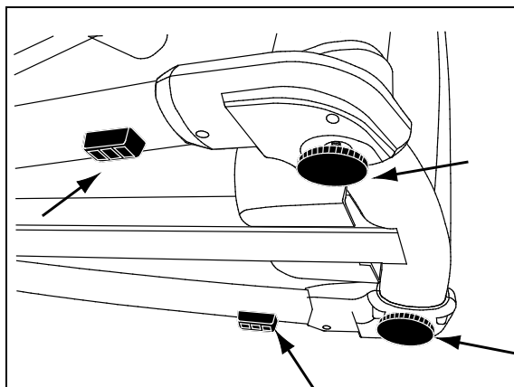
Рис. 21: Расположение резиновой подкладки и регулируемых опор
