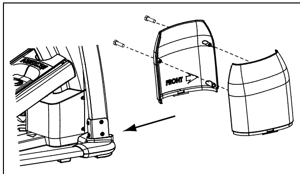
Рис. 20: Присоединение кожухов вертикальных стоек (показан правосторонний кожух)
