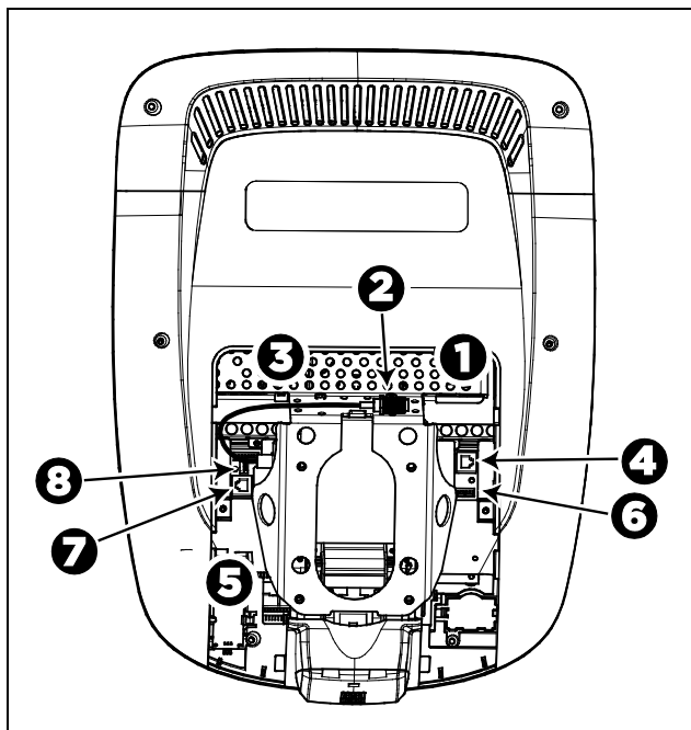
Рис. 24: Кабельные соединения, пульт P80
