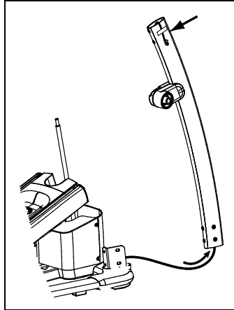
Рис. 3: Проложите кабель
