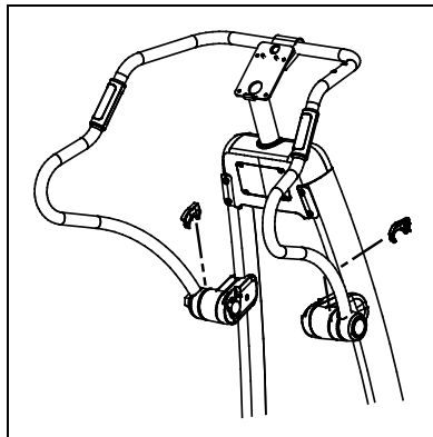
Рис. 17: Присоединение колпачков центрального перекрестия
