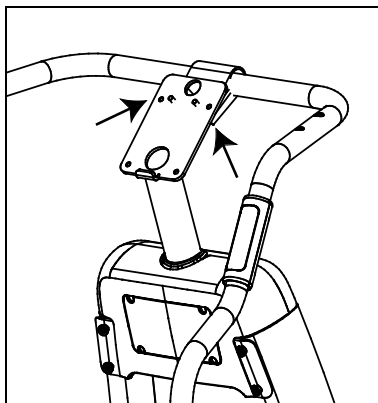
Рис. 29: Расположение винтов на скобе рукоятки
