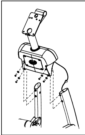
Рис. 9: Присоединение опоры центральной колонны
