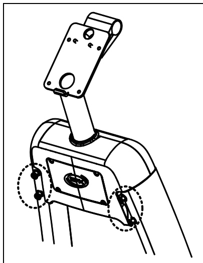
Рис. 10: Детали крепления зажима
