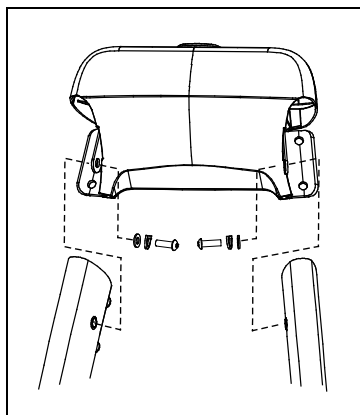
Рис. 8: Присоединение пульта, вид сзади
