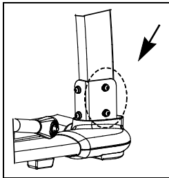
Рис. 12: Затяжка передних креплений на вертикальных стойках
