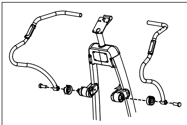
Рис. 16: Сведения о подсоединении рукояток
