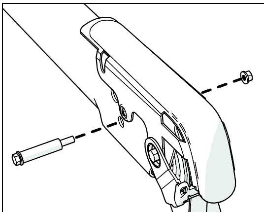
Рис.3: Крепление винта и муфты для установки боковой опоры
