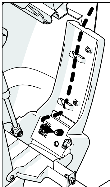
Рис.13: Прокладка кабеля в кабельном канале
