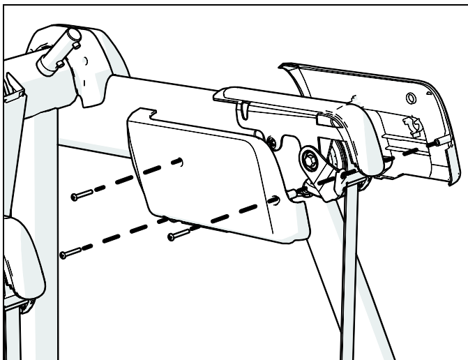
Рис.7: Установка крышек боковой опоры
