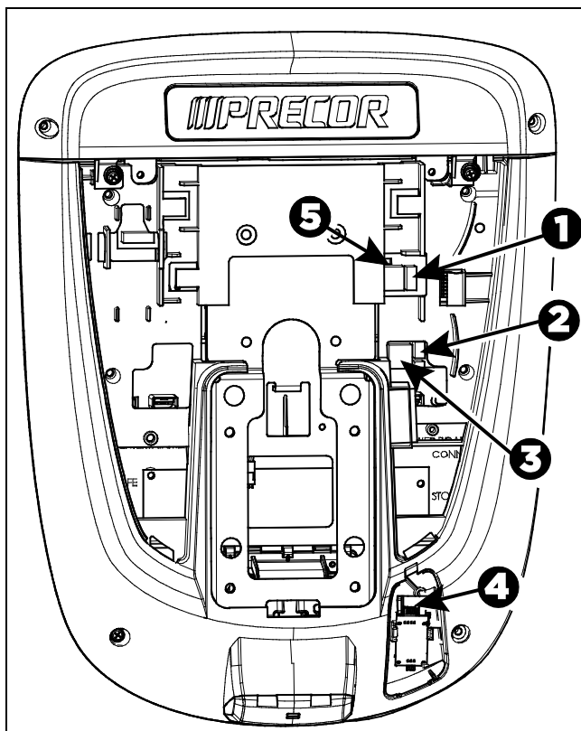
Рис.33: Разъемы кабелей, консоль P30
