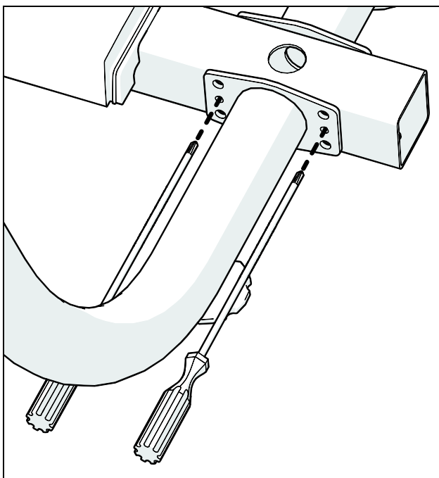
Рис.5: Выравнивание нижних боковых опор
