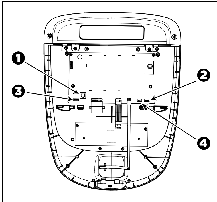
Рис.35: Подключение кабелей, пульт P20
