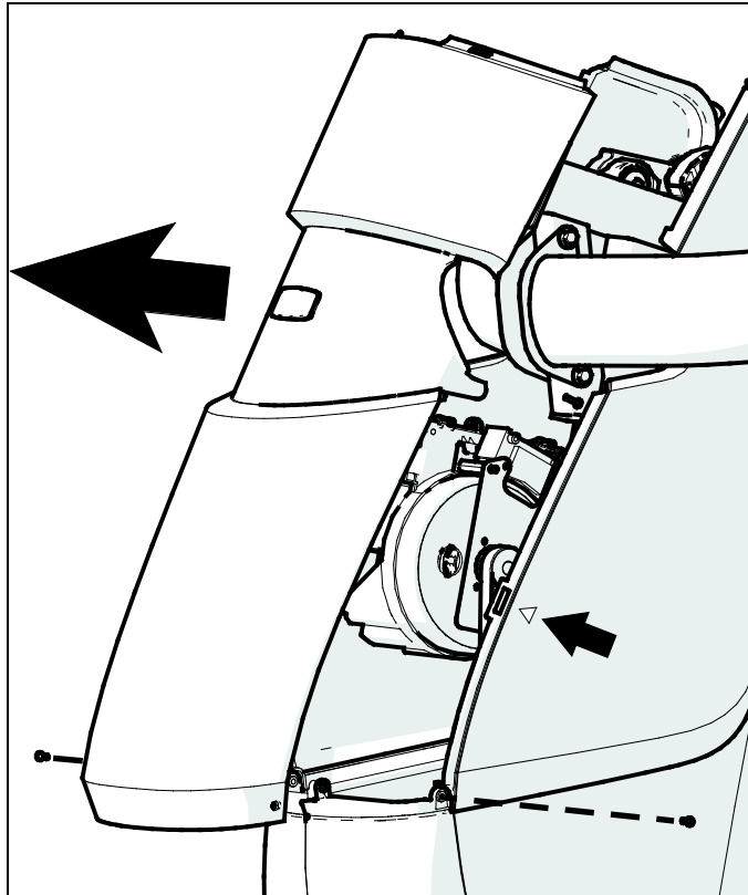
Рис.12: Снятие передней части корпуса
