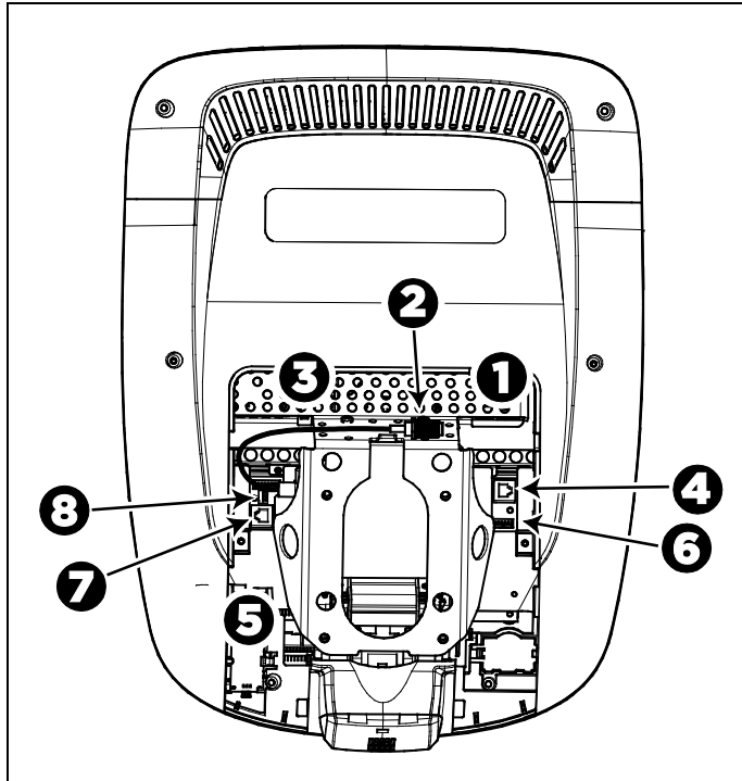
Рис.25: Кабельные соединения, консоль P80
