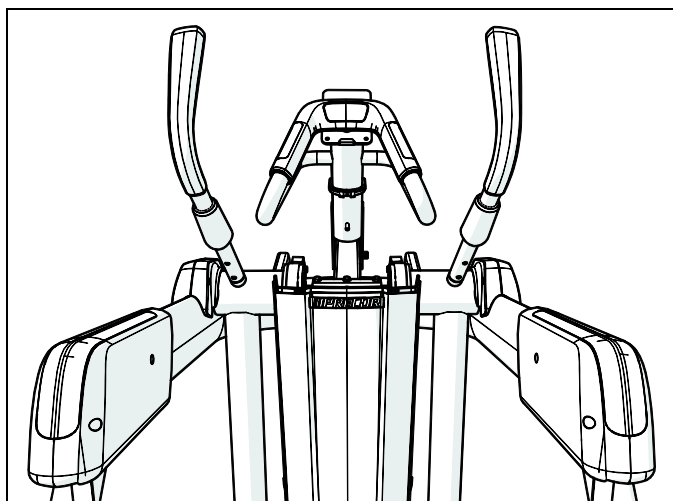
Рис.20: Установка рукояток
