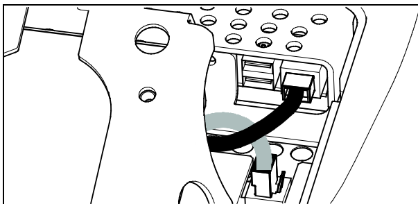
Рис.27: Подключение кабелей передачи данных Ethernet и основания аппарата
