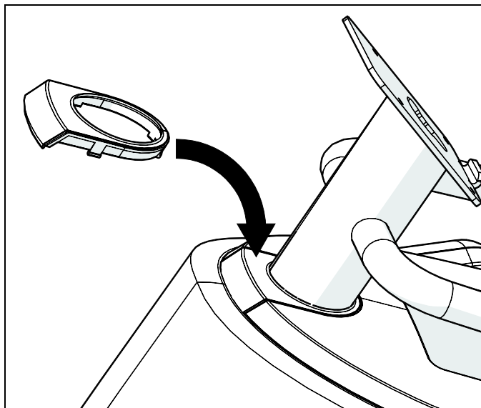
Рис.17: Установка влагоизоляции
