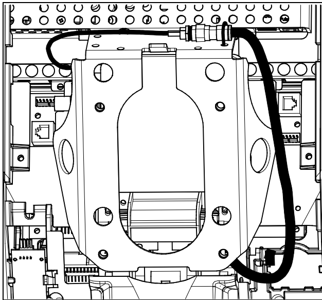
Рис.26: Подключение телевизионного кабеля
