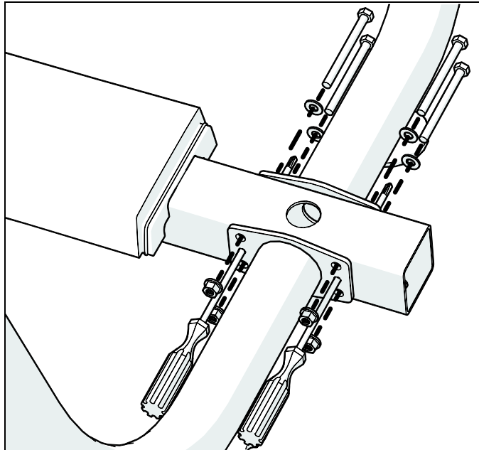
Рис.6: Установка нижних боковых опор
