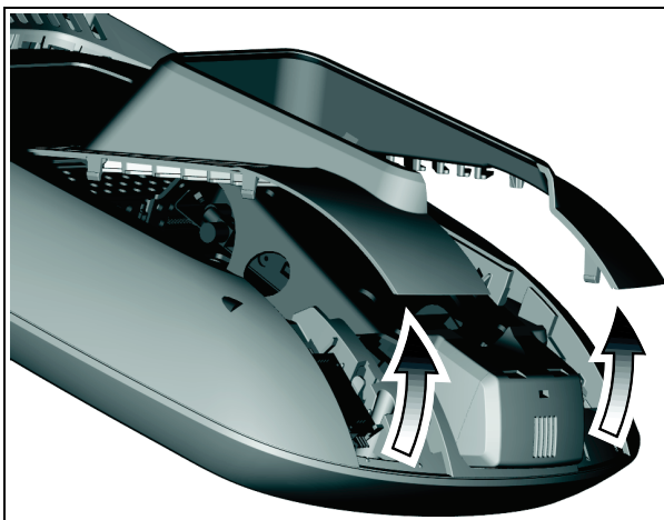
Рис.23: Снятие кожуха доступа с консоли Р80
