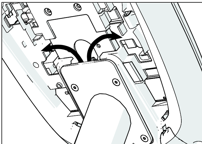
Рис.32: Прокладка кабеля из корпуса в консоль
