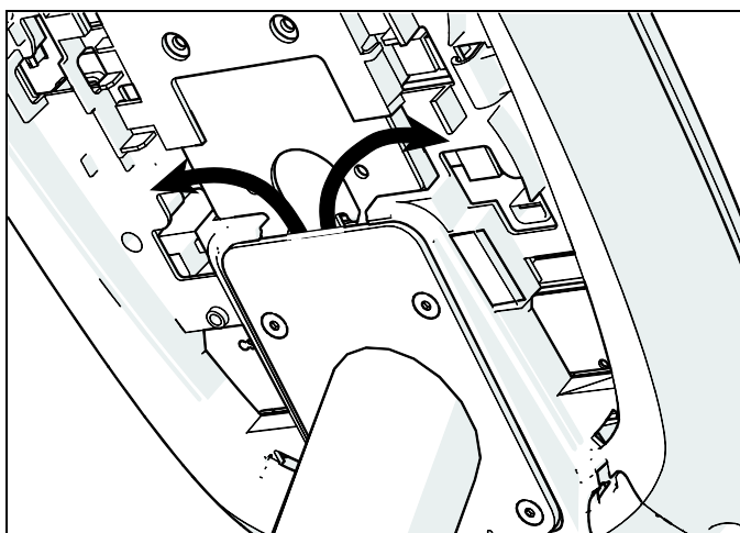
Рис.34: Прокладка кабеля из корпуса в консоль
