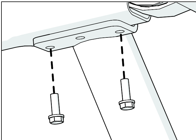
Рис.4: Установка крепежного винта на боковую опору
