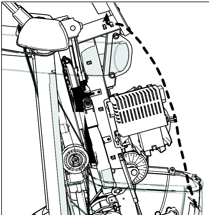
Рис.15: Прокладка кабеля вдоль рамы к центральной колонне
