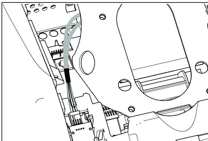
Рис.28: Подключение кабеля датчика частоты сердцебиения
