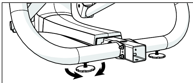
Рис.21: Расположение регулируемых опор
