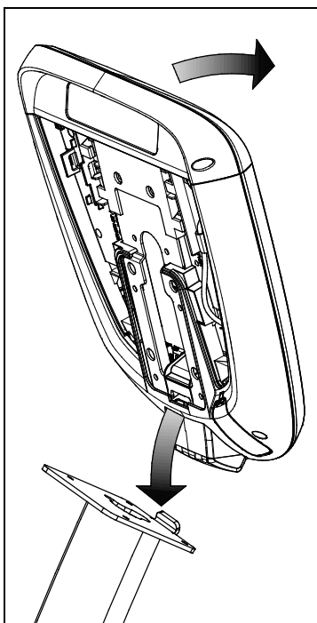
Рис.30: Размещение консоли на базе
